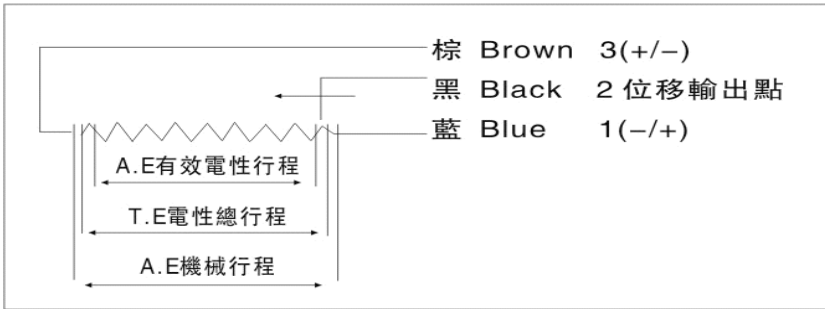
電器安裝圖
