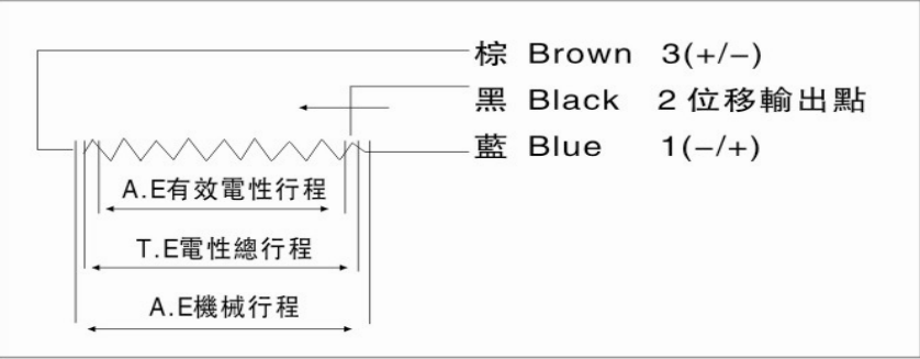
電器安裝圖
